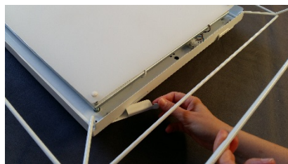
Fig. 2 Abrir los 4 pasadores de Sujeción, liberando la estructura de la base.
