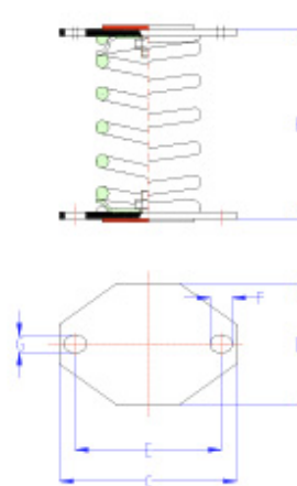
MLC-BB 150-200-250-300-350
