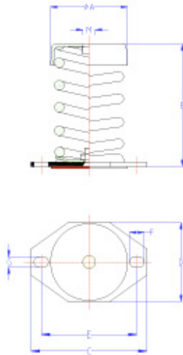
MLC-B 150-200-250-300-350
