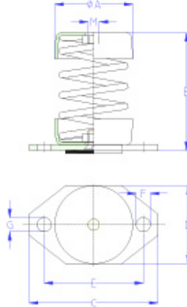
MLC-B 25-50-75-100-125
