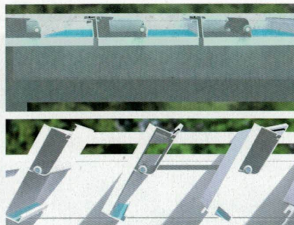
Drenaje controlado también cuando las lamas se abren
