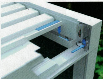
Drenaje integrado de forma eficaz
