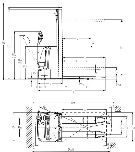
Modelos con mástiles de elevación estándar EJC 212/214/216/220
