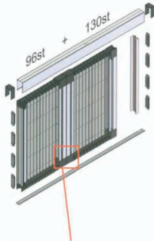
Detalle del perfil unión Detail of union profile Détail du profil union Verbindungsprofil-Detail
