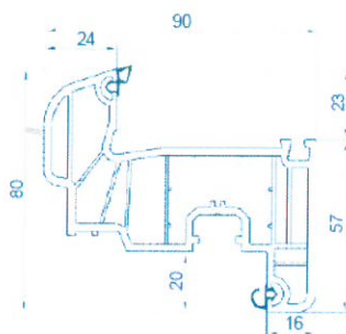
047 Hoja de 6 cámaras
