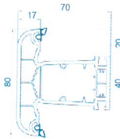
058 Intermedio de 4 cámaras
