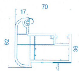
054 Perfil cierre 70 mm
