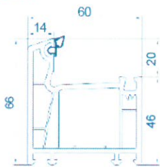
001 Marco de 4 cámaras
