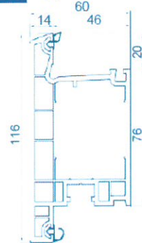
036 Hoja de la puerta (apertura exterior)
