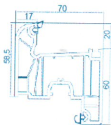
060 Hoja de 6 cámaras
