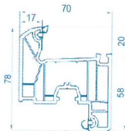
062 Hoja de 5 cámaras
