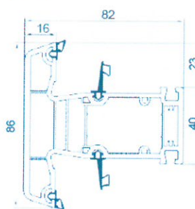
048 Intermedio de 5 cámaras
