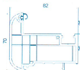
068 Perfil cierre 82mm
