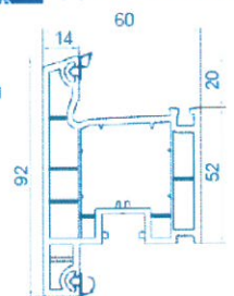
005 Hoja de la puerta (apertura exterior)
