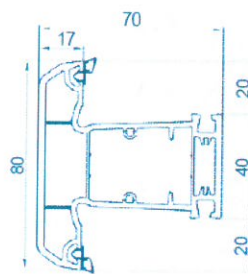
063 Intermedio de 3 cámaras
