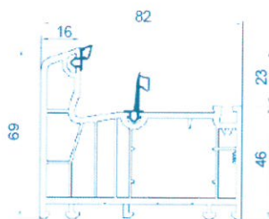
046 Marco de 6 cámaras
