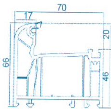
059 Marco de cámaras
