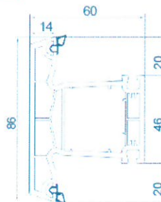
003 Intermedio de 4 cámaras
