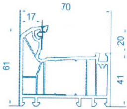
061 Marco de 5 cámaras
