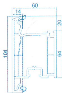
007 Hoja de la puerta (apertura exterior)
