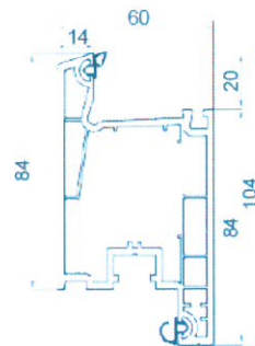
008 Hoja de la puerta (apertura interior)
