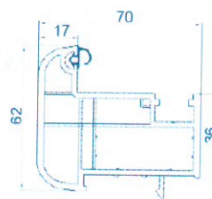
054 Perfil cierre 70mm
