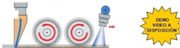
Sistema de limpieza de inyección-extracción con cepillos contragiratorios
