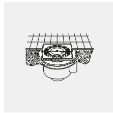
VÁLVULA OBRA 180 x 200 CON LÁMINA IMPERMEABILIZANTE
