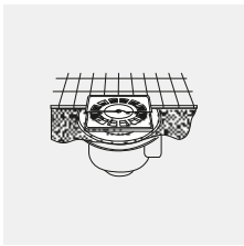
VÁLVULA OBRA 130 x 180 CON LÁMINA IMPERMEABILIZANTE
