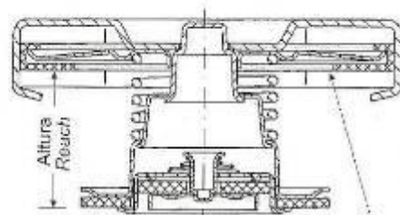
Doble junta Washer
