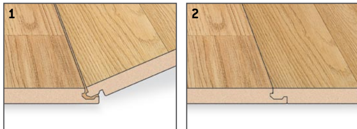
perfil longitudinal
