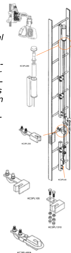
Típico Lad-Saf® Instalación Diagrama
