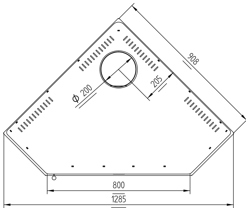
HORNO DE LEÑA MODELO HL-200 R // HL-200 RF
