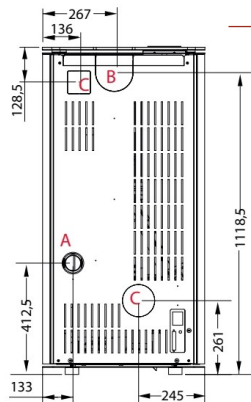
Vista laterale / Side view / Profil / Vue latérale / Seitenansicht
