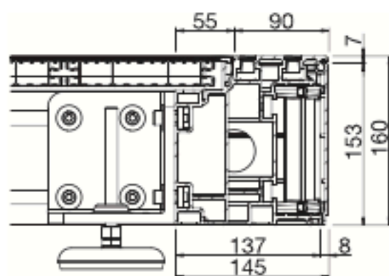
SB4700 cross-section / Sección
