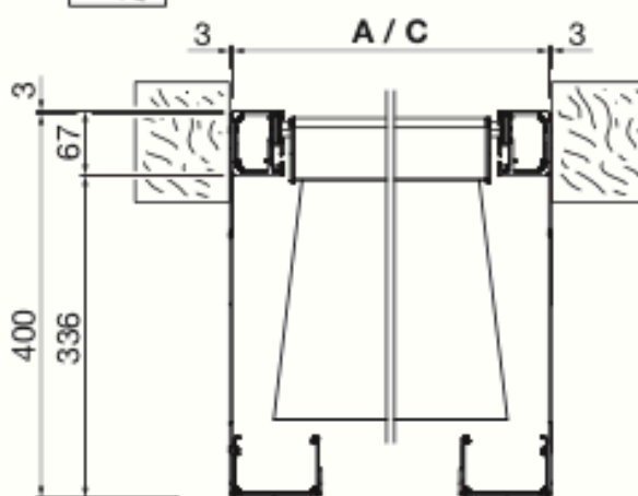
Front view incl. gutter / Vista frontal incl. canaleta de agua
