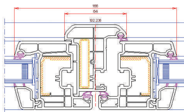
Sección Central
