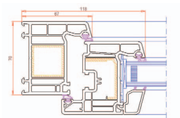
Sección Lateral
