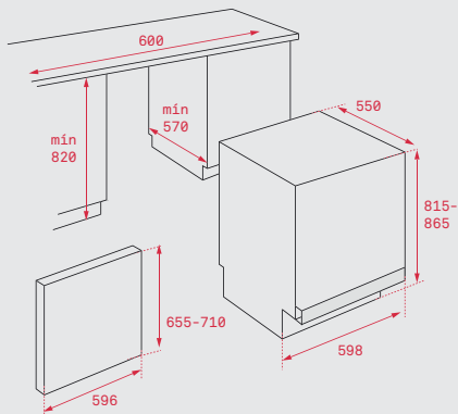
DW8 70 FI · DW8 58 FI · DW8 57 FI
