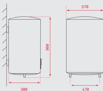
EWB 80 D SLM
