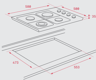
HLX 60 4G AL
