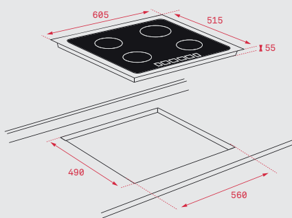
ITF 6320 · IT 6420 · IT 6350 · IT 6320 · IT 6450
