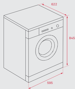
TKS 890 H · TKS1 810 H
