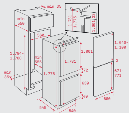
CI3 350 NF · CI3 342
