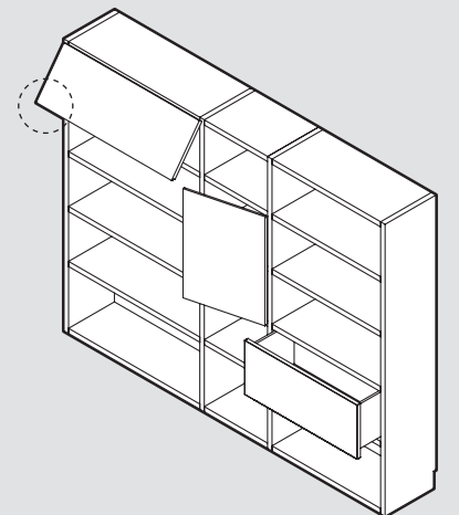
Detalle galce frentes AddBox
