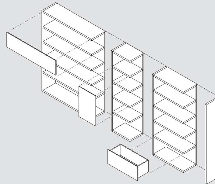
Detalle galce frentes AddBox
