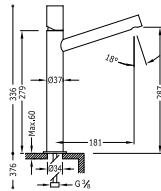
Grifo monomando XXL para lavabo Con volante. Caño largo. Latiguillos de alimentación flexibles G3/8.
