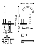
Grifo monomando de repisa para lavabo De instalación libre. Con maneta.
