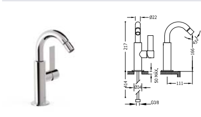
Grifo monomando con maneta lateral para bidé Rótula orientable. Latiguillos de alimentación flexibles G3/8.
