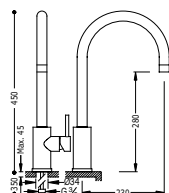
Grifo monomando para cocina Con latiguillos de alimentación flexible G3/8.
