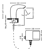
Grifo electrónico de 1 agua para lavabo Accionado mediante sensor de infrarrojos.
