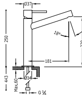
Grifo monomando alto para lavabo Con maneta. Caño largo. Latiguillos de alimentación flexibles G3/8.
