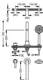
Depósito para grifería de borde de bañera (para ref.: 08115001).
