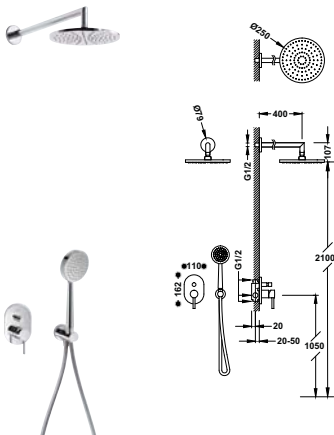
- Cuerpo empotrado incluido. - Con maneta. Inversor de 2 vías. - Brazo a pared con rociador de ducha orientable: Ø 250 mm. - Soporte para ducha de mano con toma de agua a pared. - Ducha de mano anticalcárea: Ø 100 mm. - Flexo satinado.
