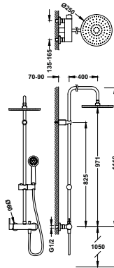
- Rociador de ducha orientable: Ø 250 mm. - Soporte deslizante y orientable para ducha de mano. - Ducha de mano anticalcárea: Ø 100 mm. - Flexo satinado.
