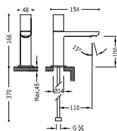
Grifo de 1 agua para lavabo Con latiguillo de alimentación flexible G3/8.
