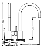
Grifo monomando para cocina Con latiguillos de alimentación flexible G3/8.
