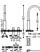
Grifo bimando alto de repisa para lavabo De instalación libre. Con volantes.
