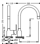
Grifo monomando con caño extraíble para cocina Con latiguillos de alimentación flexible G3/8.
