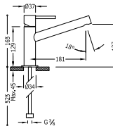
Grifo monomando para lavabo Con maneta. Caño largo. Latiguillos de alimentación flexibles G3/8.
