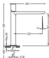
Grifo monomando XXL para lavabo Con volante. Latiguillos de alimentación flexibles G3/8.
