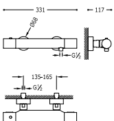
Grifo termostático mural para ducha Ducha de mano anticalcárea. Soporte orientable para ducha de mano. Flexo satinado.
