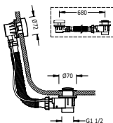
Válvula de desagüe automático para bañera con rebosadero Con rebosadero. Tapón: Ø 43 mm. Tubo flexible: máx. 680 mm.
