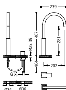
Grifo monomando alto de repisa para lavabo De instalación libre. Con maneta.
