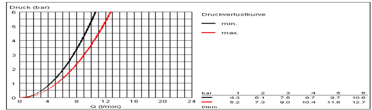
13950-13951 (Con limitador)
