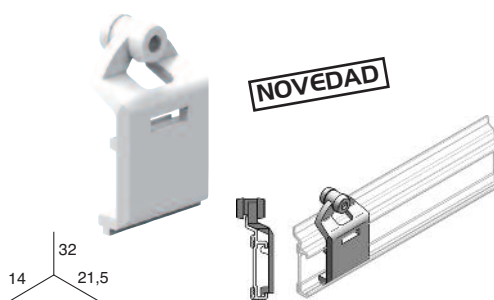
CORREDERA CON RUEDA
