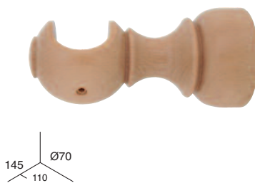
SOPORTE ABIERTO
