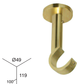
SOPORTE TECHO ABIERTO LARGO (No disponible en dorado y bronce satinado)
