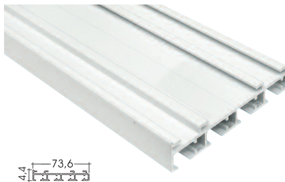
PERFIL 4 VÍAS
