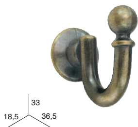
GANCHO LISO (No disponible en blanco)
