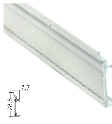
PERFIL PORTATELA
