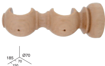
SOPORTE ABIERTO DOBLE 35-35
