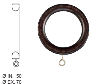
ANILLA "LISBOA"
