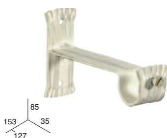
SOPORTE LARGO
