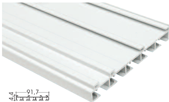
PERFIL 5 VÍAS
