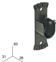
SOPORTE LATERAL ABIERTO
