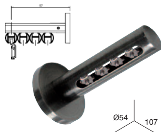
SOPORTE MÚLTIPLE (x4)
