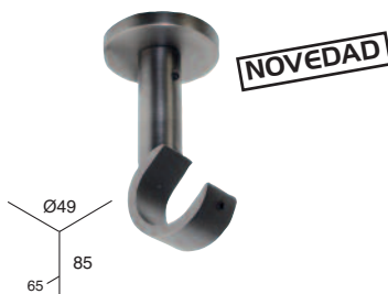
SOPORTE TECHO ABIERTO CORTO (No disponible en dorado y bronce satinado)
