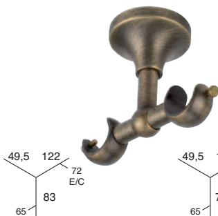
SOPORTE TECHO DOBLE
