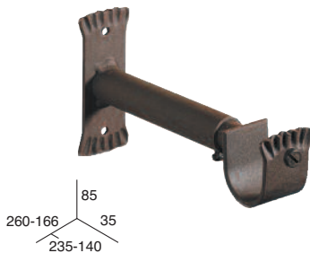
SOPORTE EXTENSIBLE
