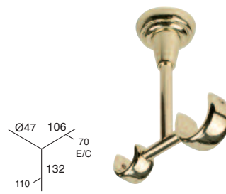
SOPORTE TECHO DOBLE 28-20 mm. (No disponible en níquel negro y titanio mate)
