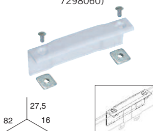
UNIÓN MANGUITOS PORTA-POLEAS P-900 Y 910 (para porta-poleas 7297060 y 7298060)
