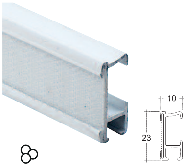
PERFIL 942
