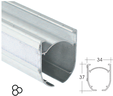
PERFIL 7347
