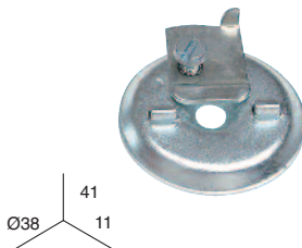
SOPORTE TECHO ARTICULADO
