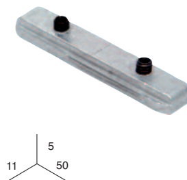
EMPALME (perfil 950/910)
