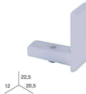
TAPÓN PERFIL
