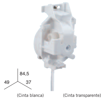
CARRETE CON CINTA 2,40 m.
