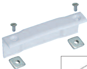
UNIÓN MANGUITOS PORTA-POLEAS P-900 Y 910 (para porta-poleas 7297060 y 7298060)
