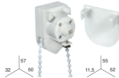
EMBRAGUE 1:2 + TAPÓN CON CADENILLA
