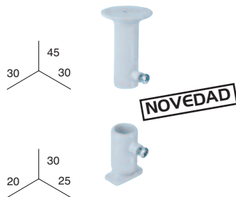
ACCESORIO PARA SOPORTE TECHO "CHYC"
