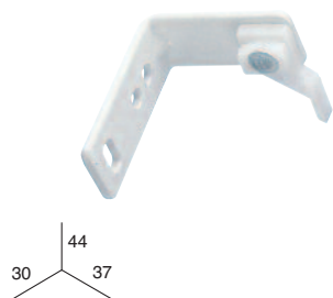
SOPORTE 3 cm.
