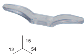
CORNAMUSA. TRANSPARENTE
