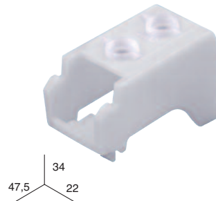
SOPORTE FRENTE TECHO
