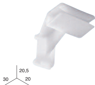
SOPORTE PERFIL 7206 A PERFIL 1078
