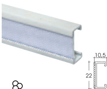
PERFIL 7206
