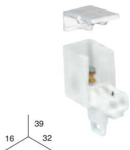
PORTA-POLEAS RETORNO
