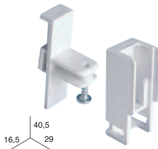
SOPORTE LATERAL
