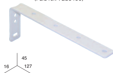
SOPORTE FRENTE 12 cm. (Para ref. 7286400)
