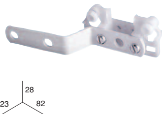
CORREDERA MAESTRA CON RUEDA Y PATA CORTA (recomendada para riel con curva)
