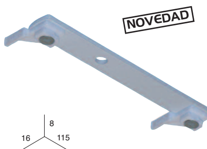
PLETINA DOBLE TECHO 100
