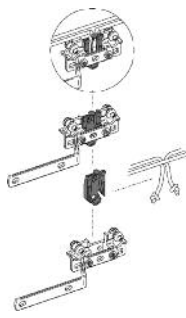
BRIDA CORDÓN
