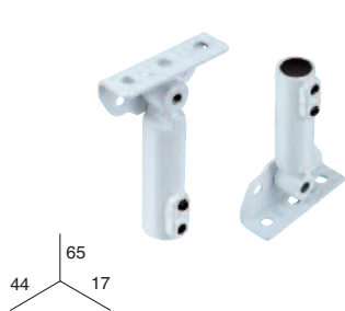
CASQUILLO RIOSTRA (Para perfiles 900, 908, 910 y 950)
