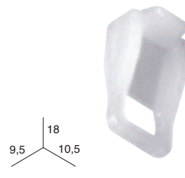
CORREDERA SIMPLE
