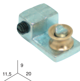
POLEA INTERMEDIA
