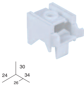
SOPORTE FRENTE-TECHO
