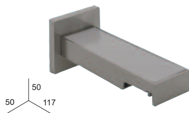
SOPORTE DECORATIVO
