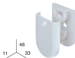
DISPOS.SEGURIDAD CADENILLA. BLANCO
