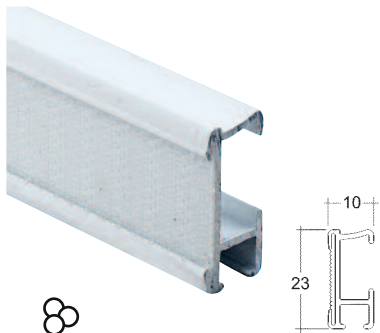
PERFIL 942
