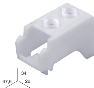
SOPORTE ESTOR FRENTE-TECHO LARGO
