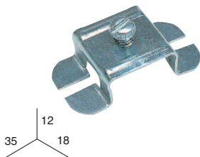
ESTRIBO FRENTE (Para refs. 7187060 y 7188060)
