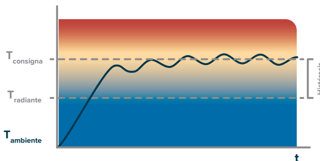
Sistemas Airzone con control de la inercia térmica
