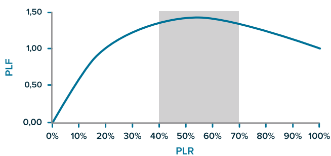
RANGO DE FUNCIONAMIENTO DE ECO-ADAPT EN UNA MÁQUINA INVERTER
