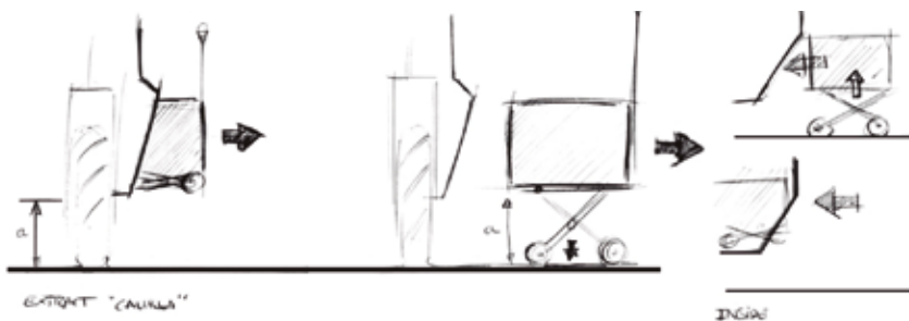
Primeros bocetos sistema de extracción del Power Battery Pack en 2012
